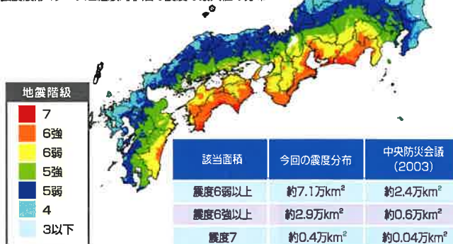
【震度の最大値の分布図】 強震波形4ケースと経験的手法の震度の最大値の分布
